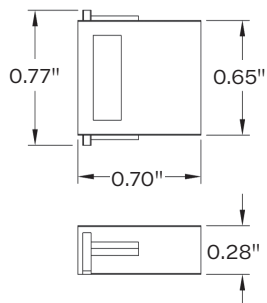
RGBW end cap
